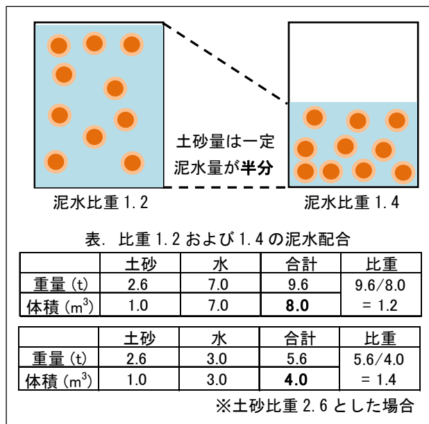
図-2 比重 1.2 と 1.4 の泥水の体積比較
