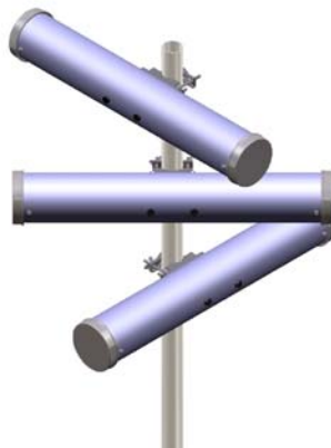
図3 円偏波型アンテナ
