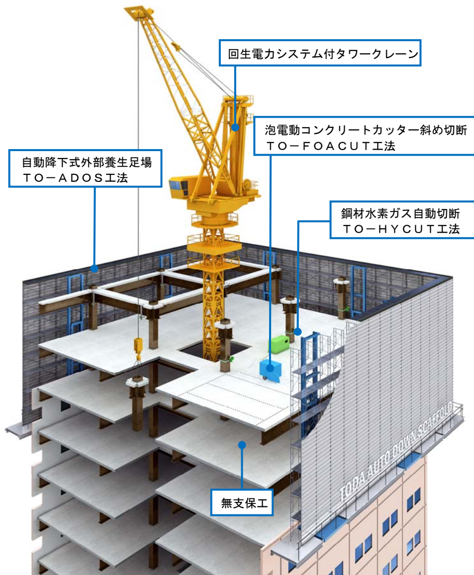
図1 超高層解体工法TO-ZERO模式図
