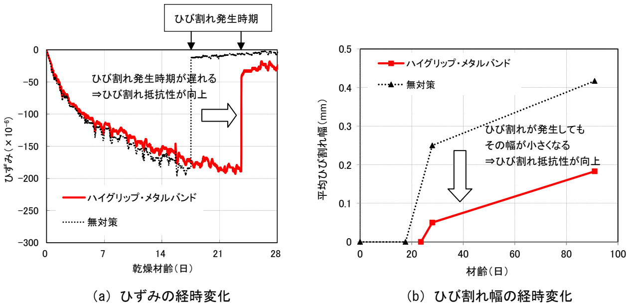
図-1 拘束されたコンクリートの乾燥収縮ひび割れ試験結果
